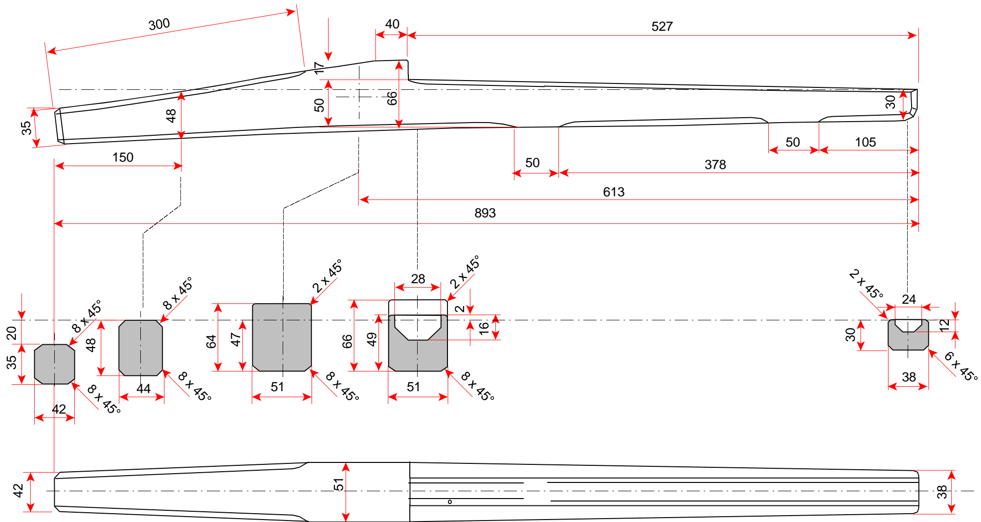
Frühes Luntengewehr, um 1450 Schaft
